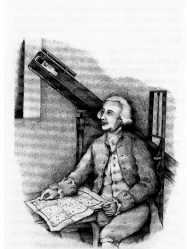
युरेनसचा शोध लावताना हर्षल व त्याची दुर्बीण
